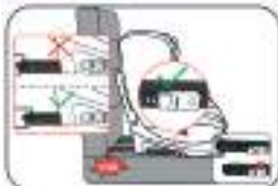
Βήμα 3. Εισαγάγετε το ISOFIX του βρεφικού καθίσματος στο αντίστοιχο σταθερό σημείο ISOFIX του αυτοκινήτου και θα ακουστεί ένα κλικ εμφανίζοντας παράλληλα ένα πράσινο σημάδι στο σχετικό παράθυρο. Μέχρι να τοποθετηθεί σωστά το ISOFIX, το παράθυρο θα εμφανίζει κόκκινο χρώμα.
