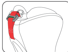
Βήμα 4. Όπως φαίνεται στην εικόνα, πριν από την τοποθέτηση του ISOFIX, βγάλτε το κει του άνω μιάνα πρόσδεσης στο πίσω κάλυμμα, τραβήξτε προς τα έξω τον μάντα επεκτείνοντας τον και κρεμάστε τον προσωρινά στην κεφαλή του καθίσματος.
