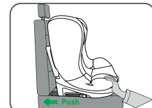
Βήμα 4. Πιέστε το παιδικό κάθισμα στο πίσω μέρος του καθίσματος του αυτοκινήτου ώστε να εφαρμοστεί στεθερά. Αντικινήστε το κάθισμα από πλευρά σε πλευρά για να βεβαιωθείτε ότι είναι σωστά στερεωμένο.
